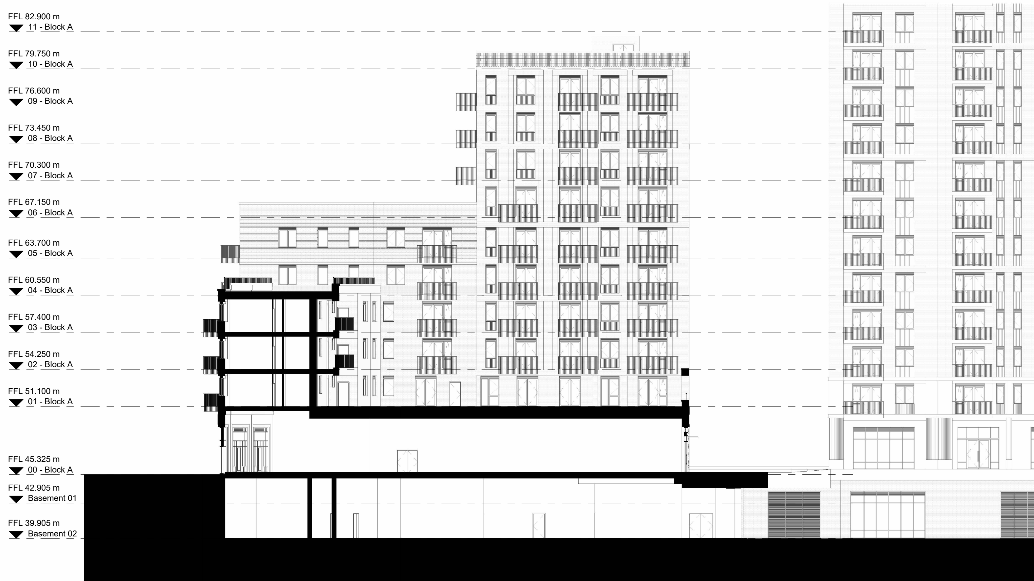
Block A - Section DD 1 : 200
