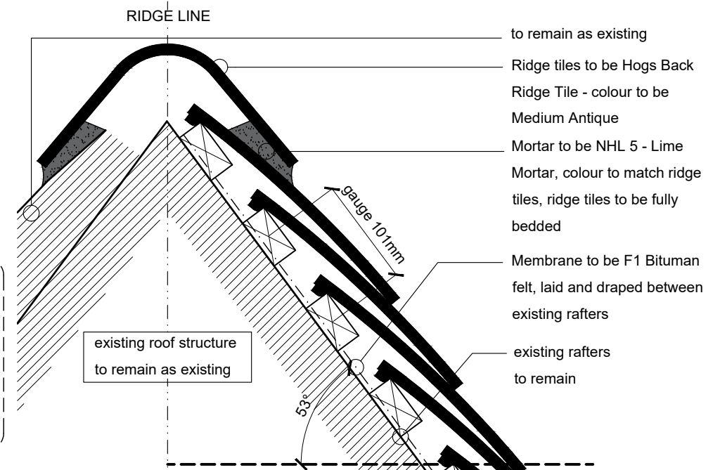
02 Ridge Detail 02 Scale: 1:5
