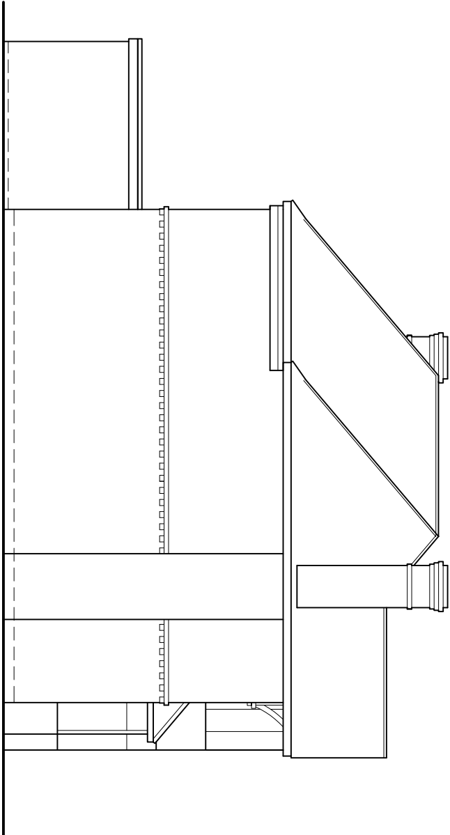
L.H. side elevation
