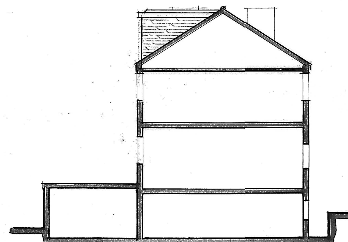
Flank Elevation
