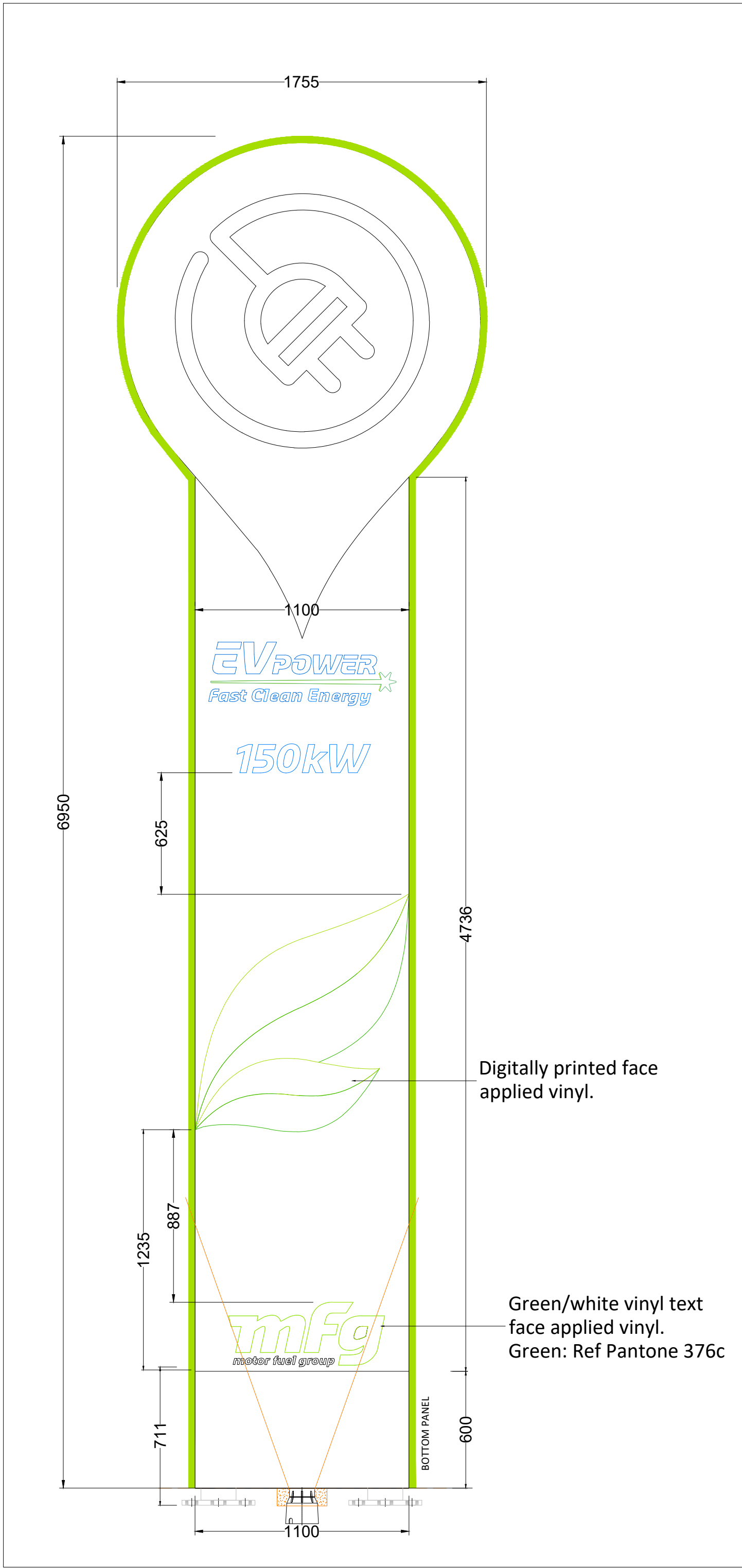
7M EV POLE SIGN Scale: 1:20
