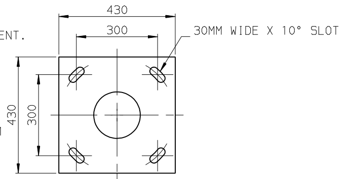
FLANGE PLATE OPTION SCALE: 1:10
