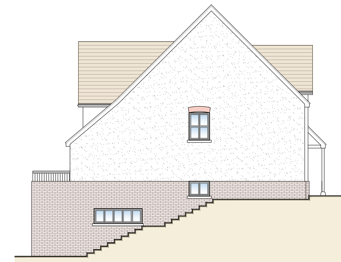
SIDE ELEVATION - PLOT-1,2
