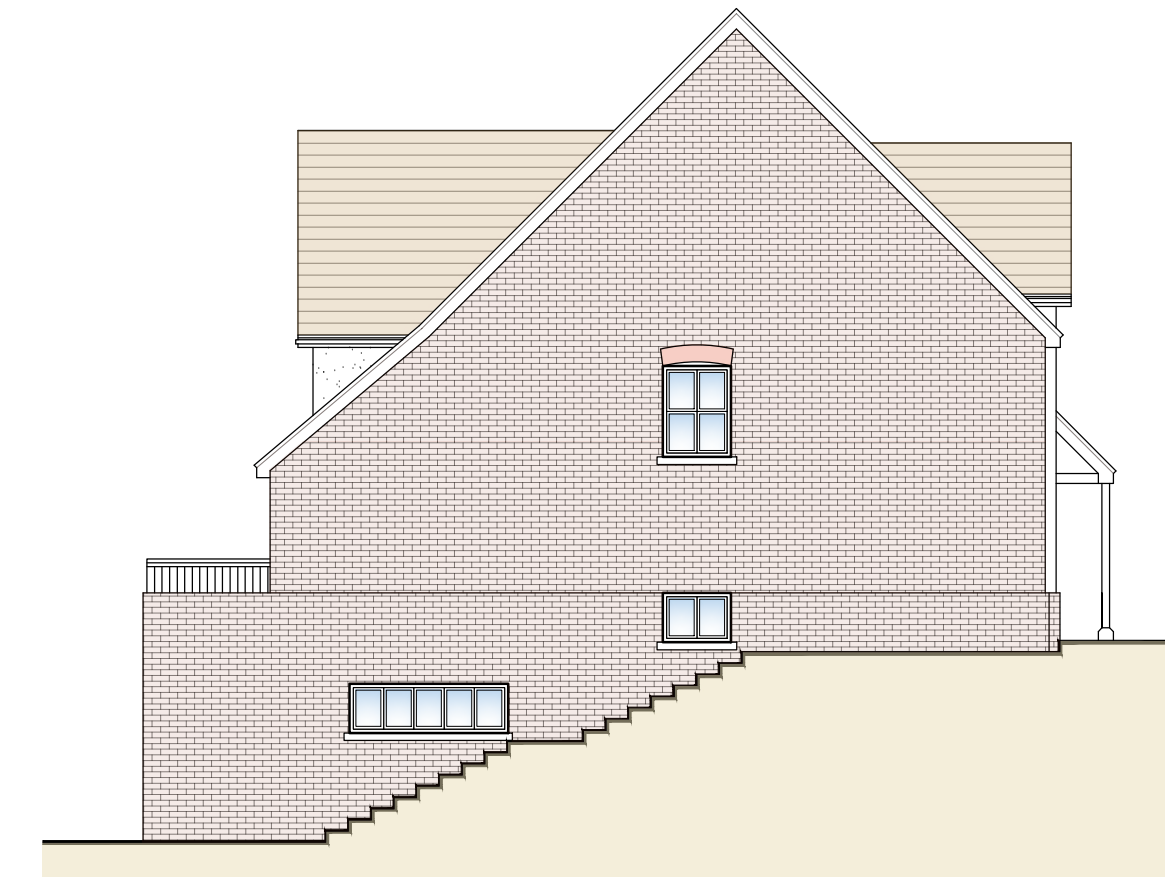
SIDE ELEVATION - PLOT-3,4
