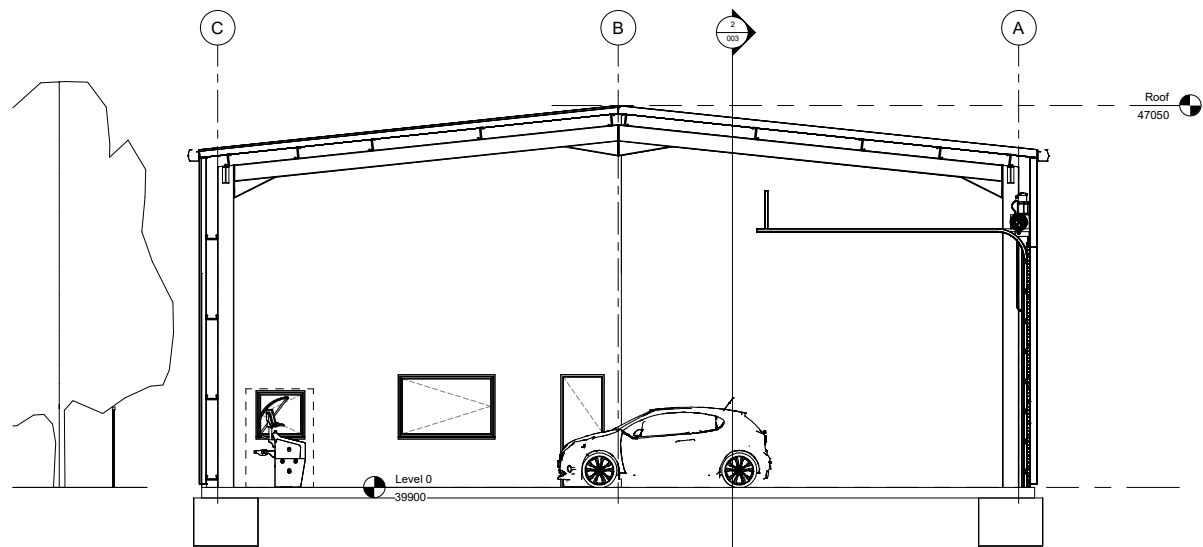
1 Section 1-1 1 : 50
