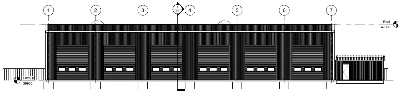
② East 1 : 100
