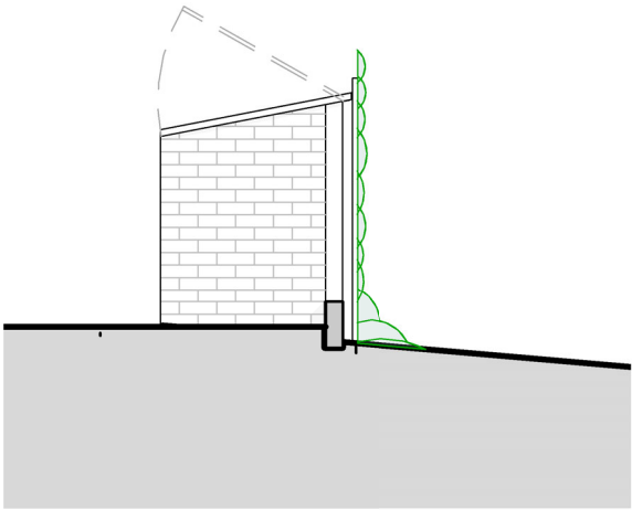
Bike Store Side - SE 1 : 50
