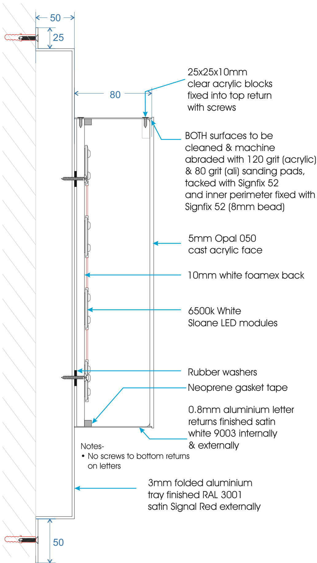
Scale 1:3
