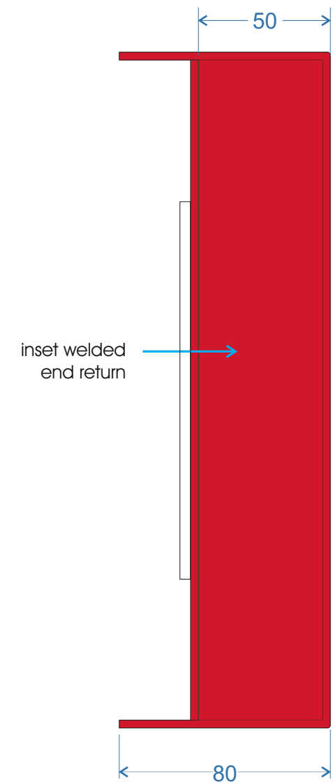
Scale 1:2
