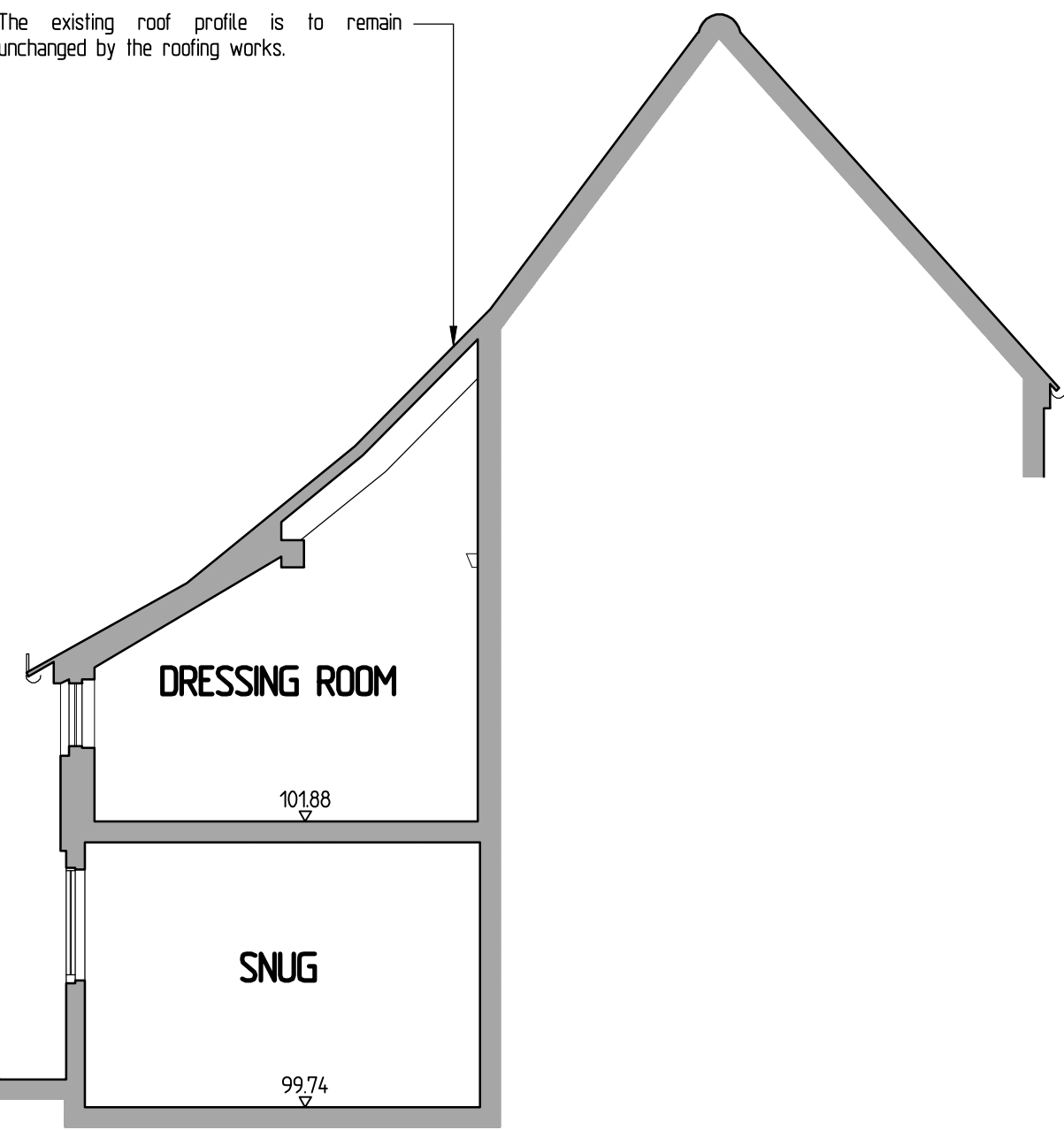
Section A-A - 1:50
