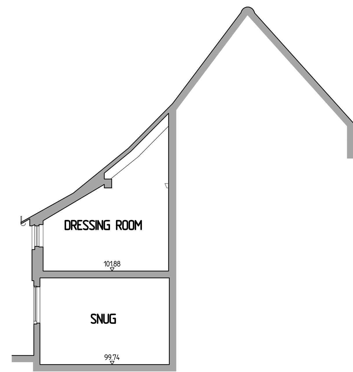
Section A-A - 1:50
