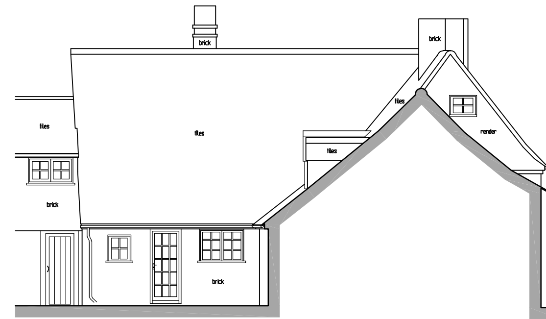
Side (S.W.) Elevation - 1:100
