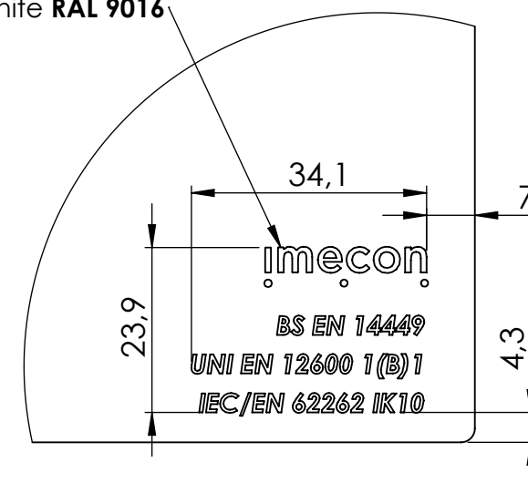
DETAIL D SCALA 1 : 1
