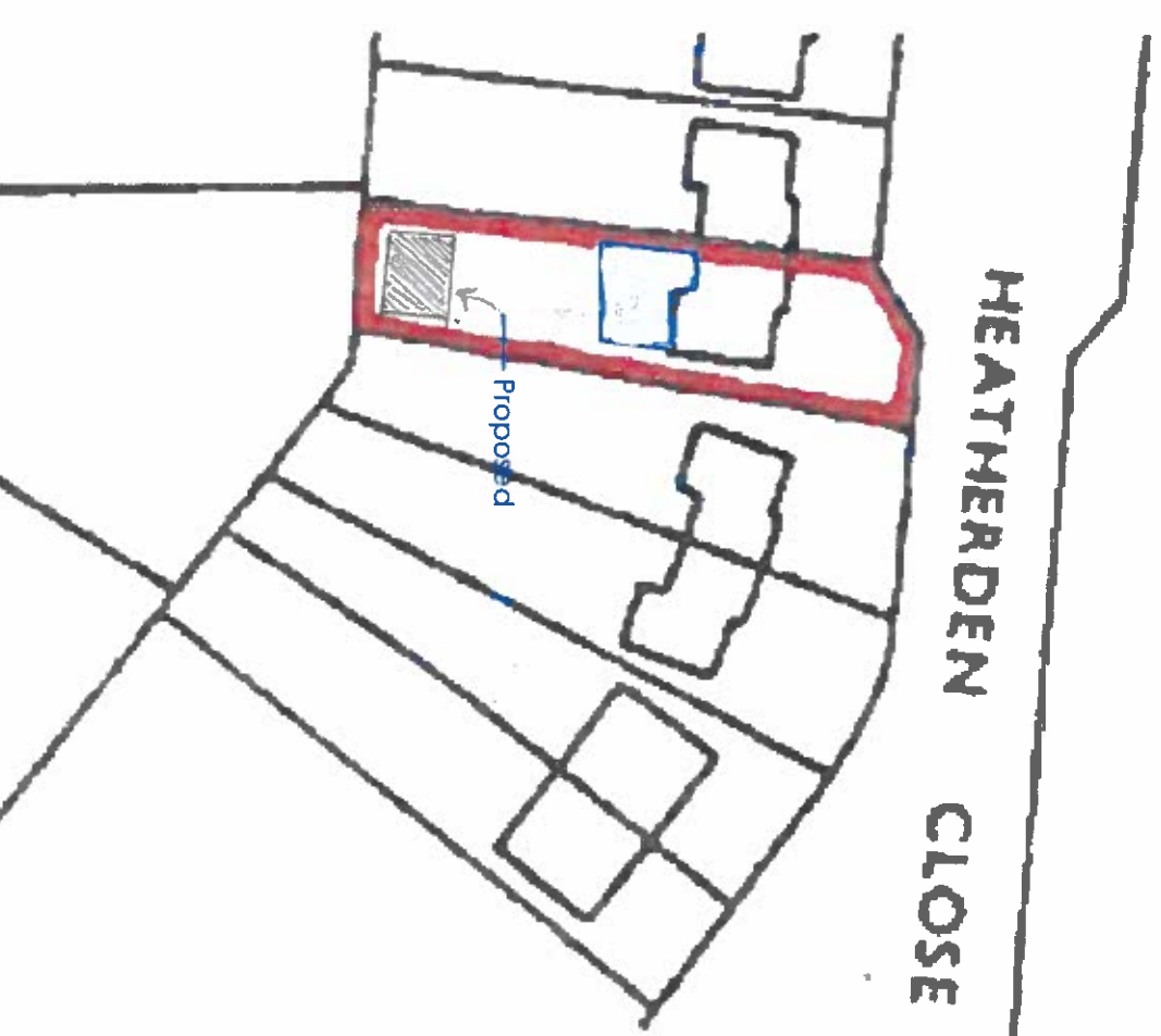
Site plan 1 / 500
