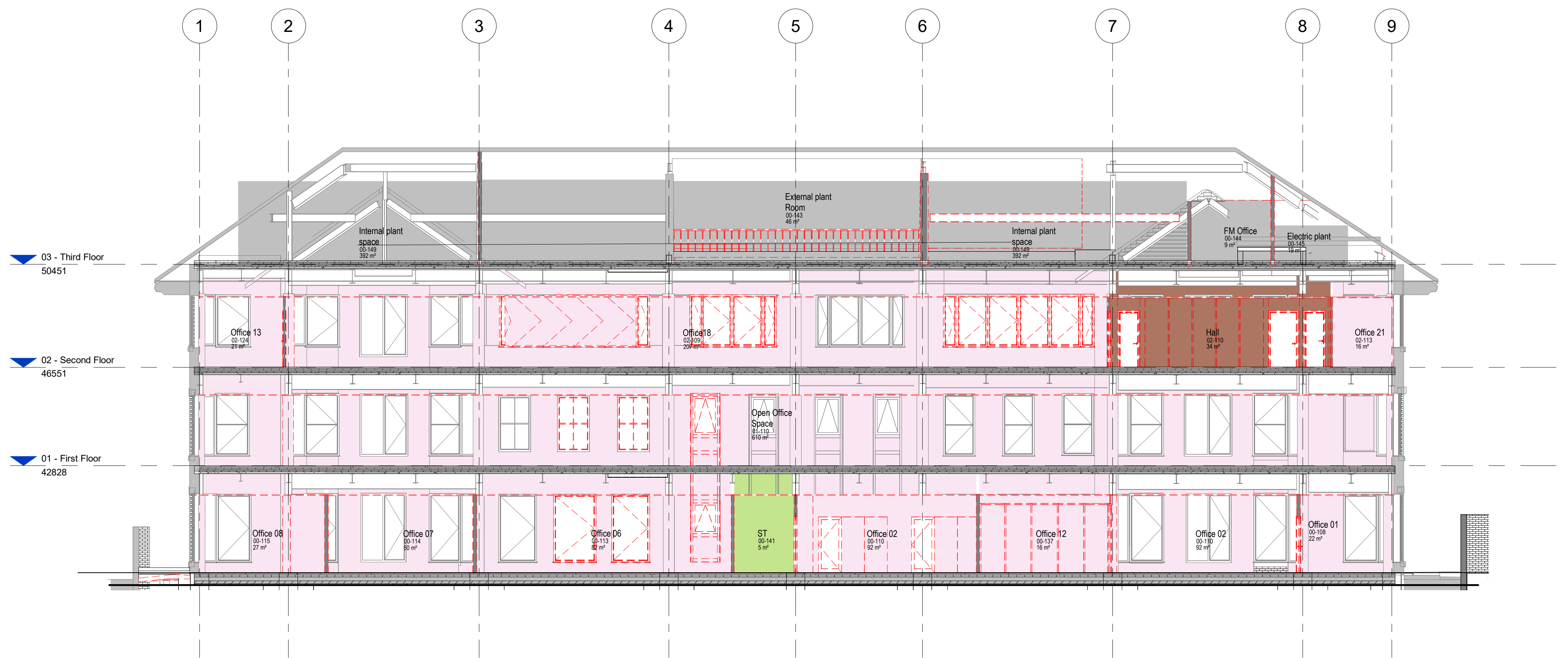
Existing section A - A 1 : 100
