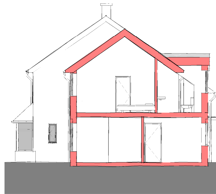
7 Section 1 : 100
