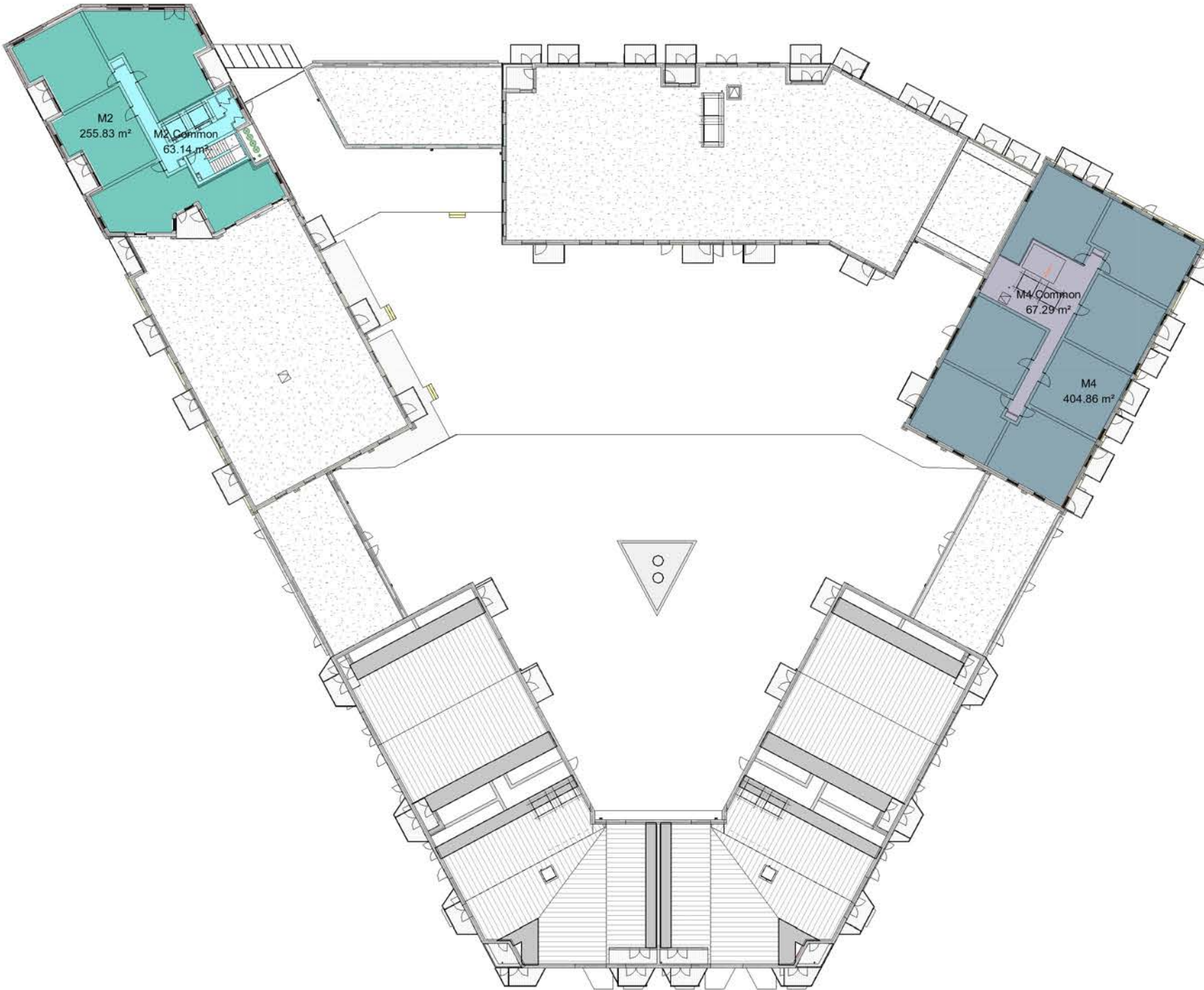
Level 7 1 : 500
