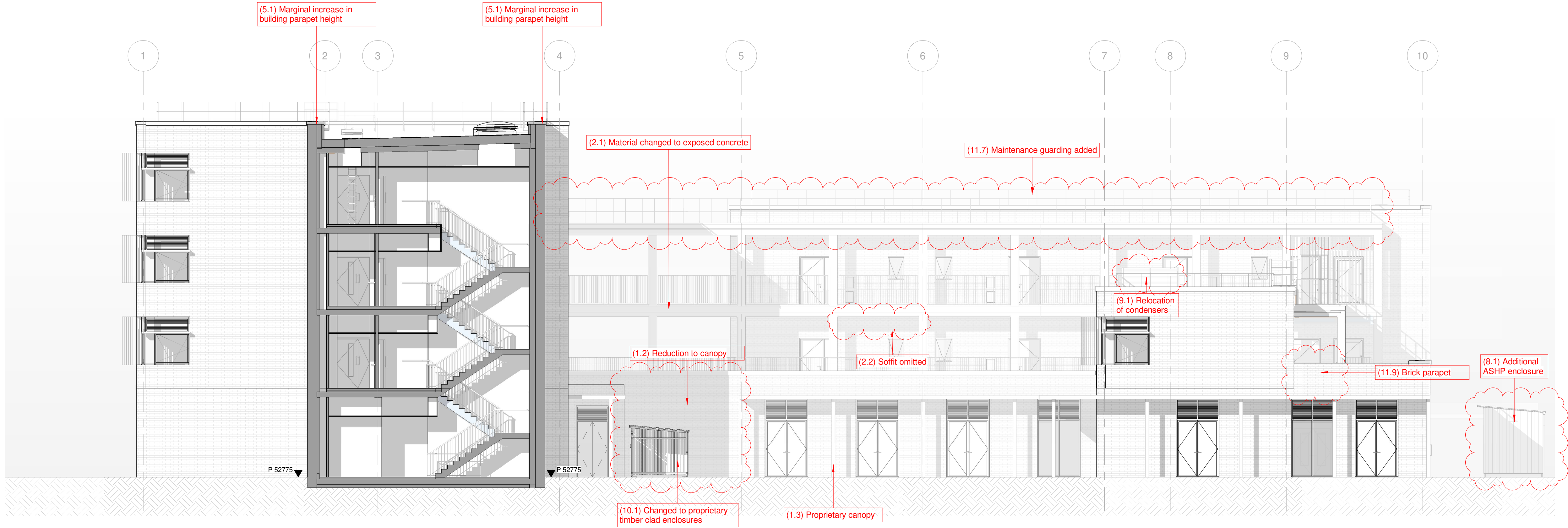
A GA Section 03 1 : 100
