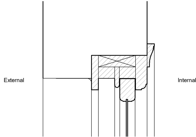
4 Window jamb detail 1 : 5
