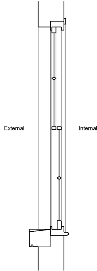
2 Section 1 : 20
