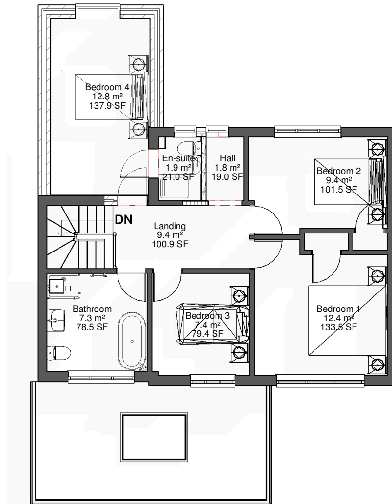
2 Level 1. 1 : 100
