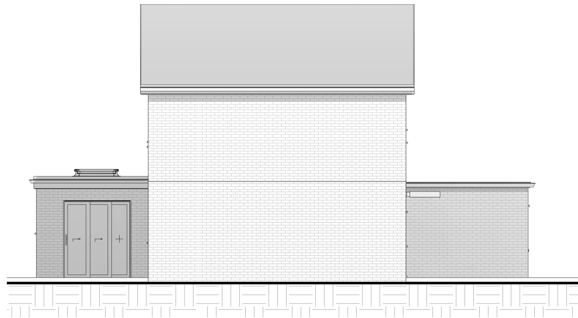
2 East 1 : 100
