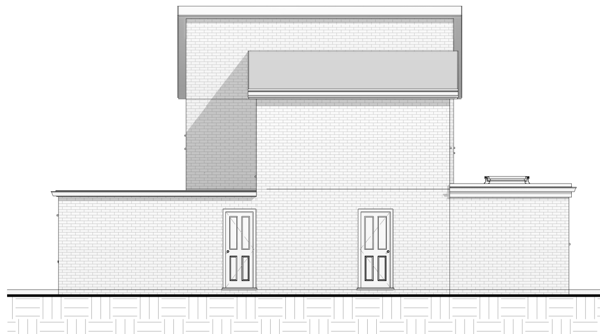
4 West 1 : 100
