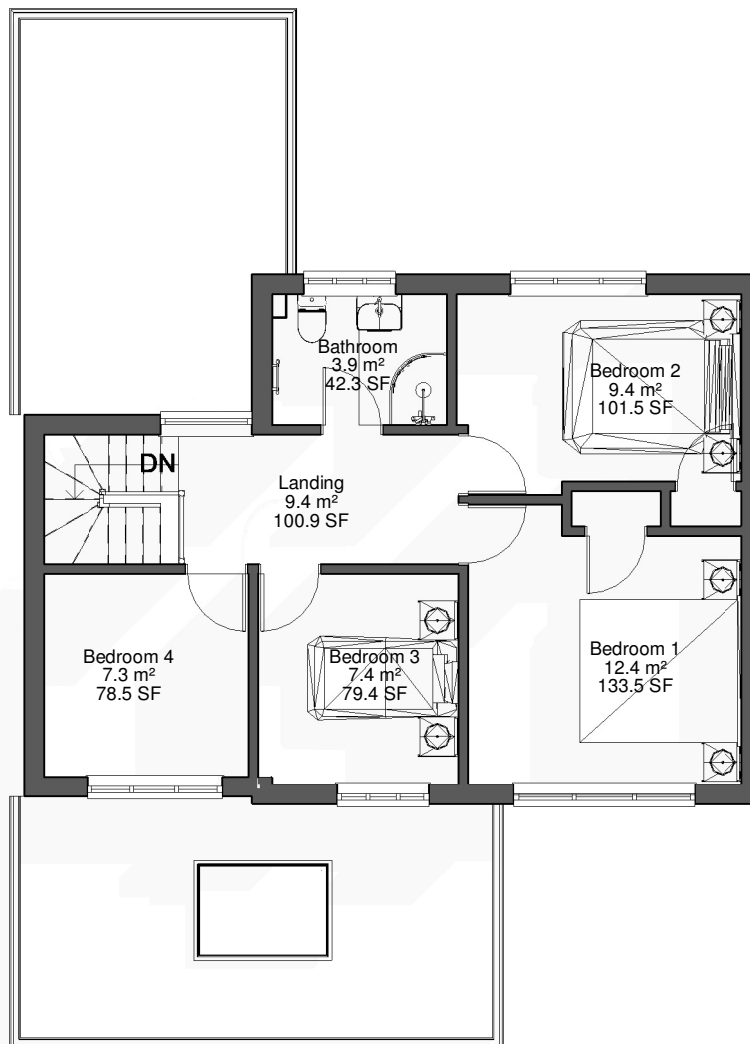
2 Level 1 1 : 100
