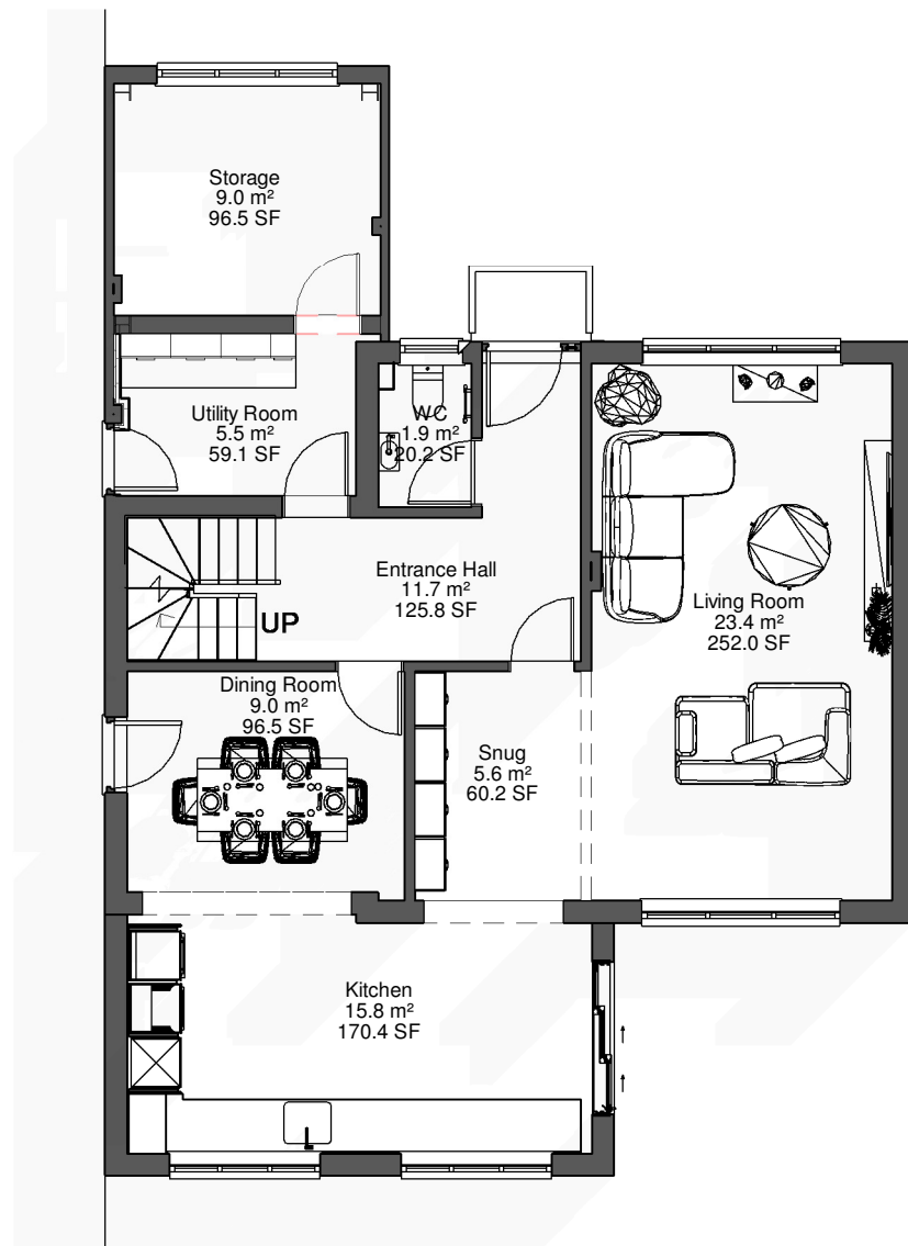
1 Level 0. 1 : 100
