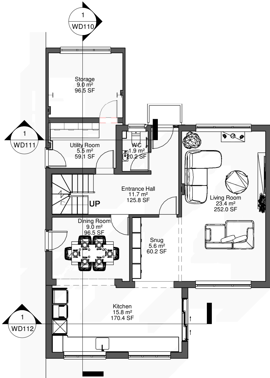
1 Level 0. 1 : 100
