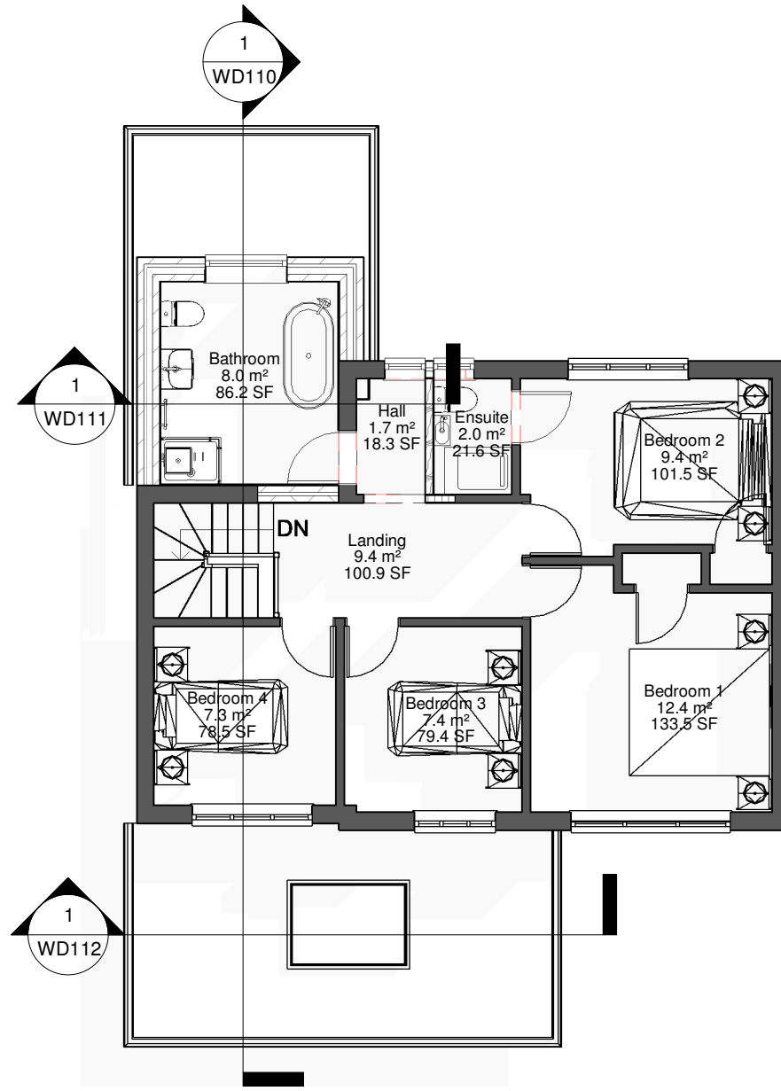
2 Level 1. 1 : 100
