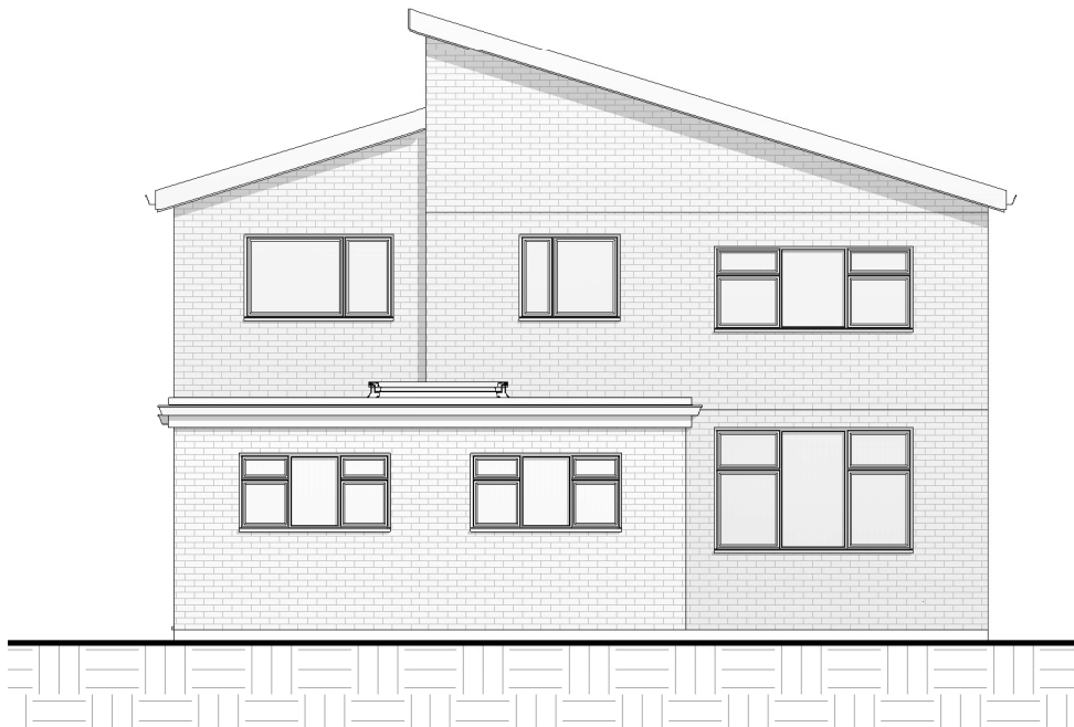
3 East 1 : 100
