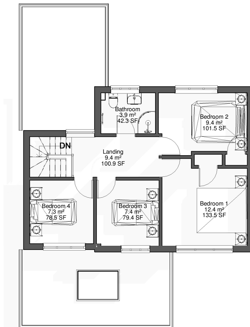
2 Level 1 1 : 100
