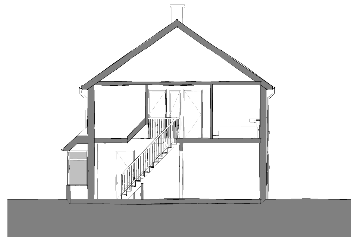
4 Section A 1 : 100
