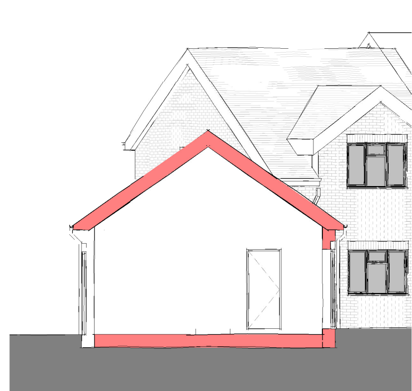
9 Section C 1 : 100
