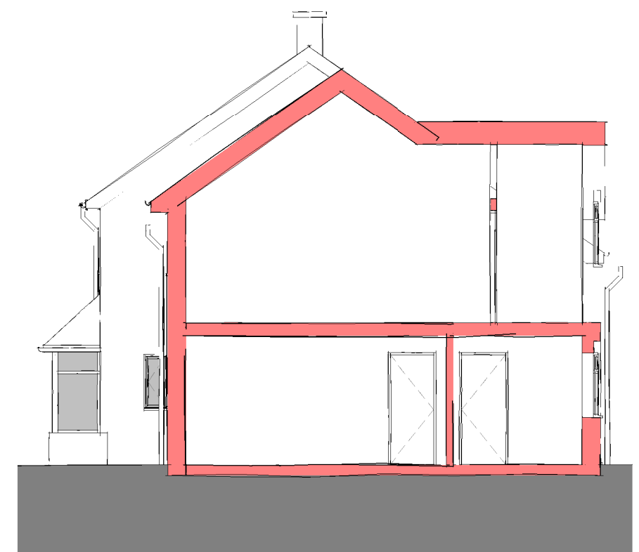
8 Section B 1 : 100
