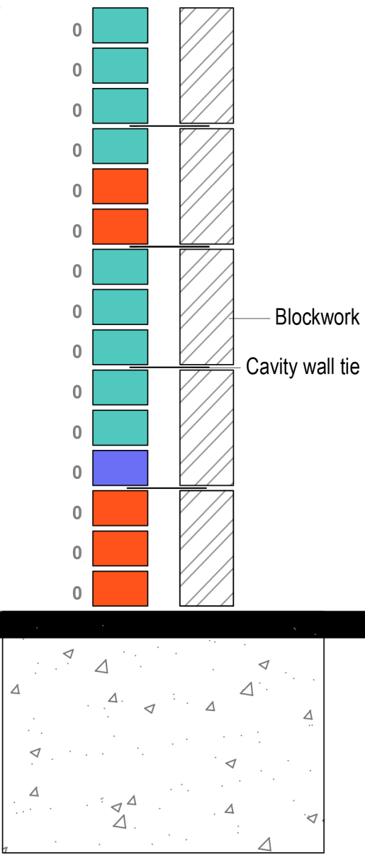
Section A-A
