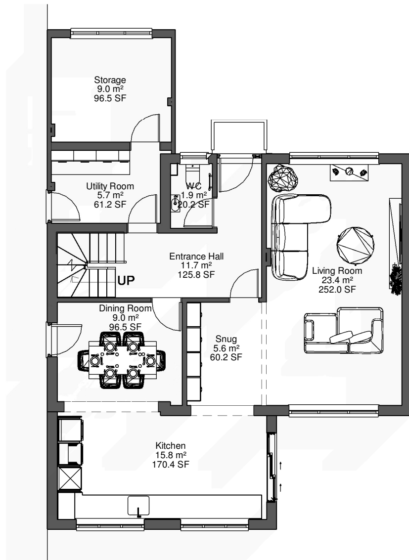
1 Level 0. 1 : 100
