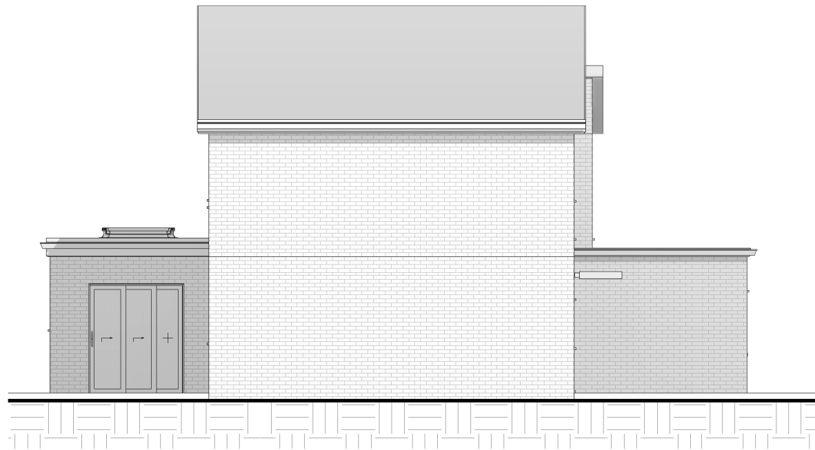
2 East. 1 : 100
