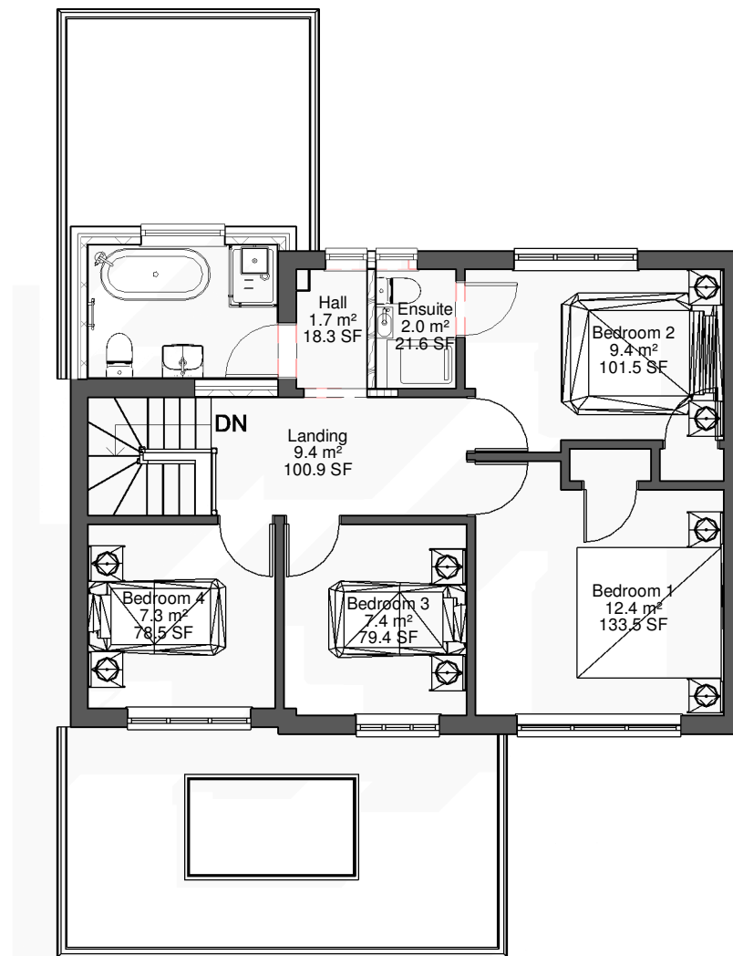
2 Level 1. 1 : 100
