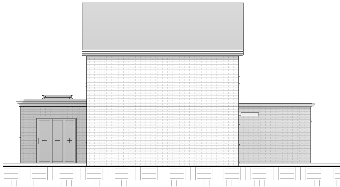
2 East 1 : 100
