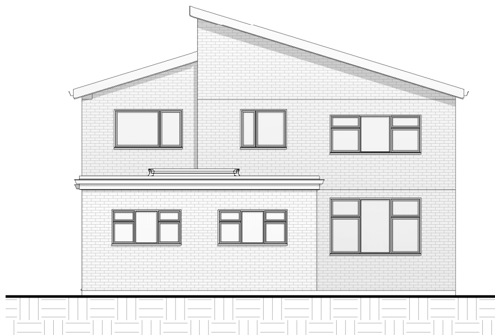
3 South 1 : 100
