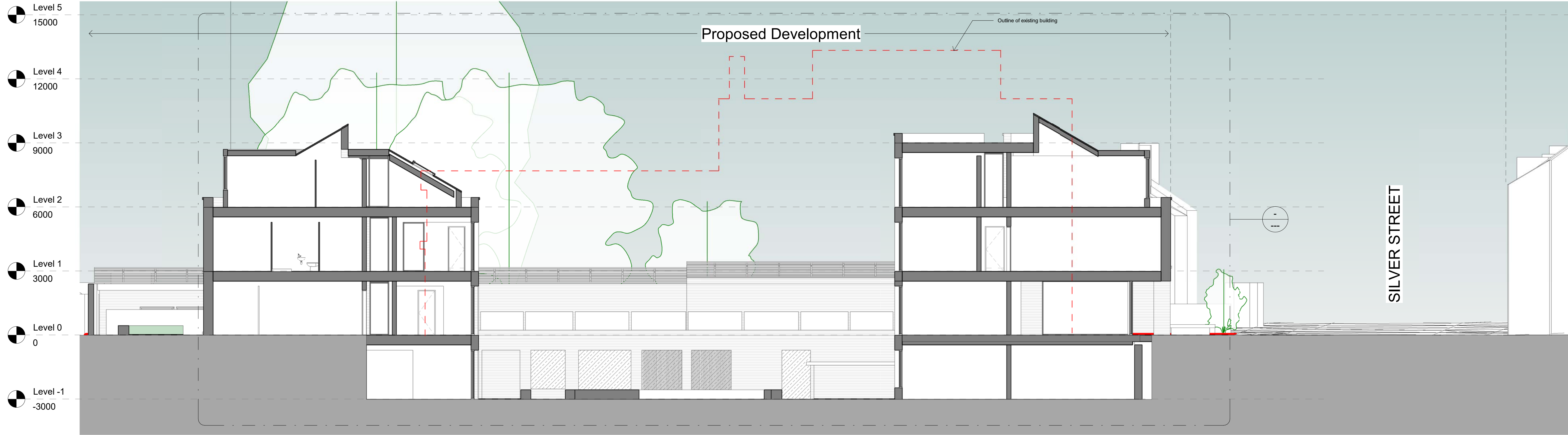
Section DD 1 : 100
