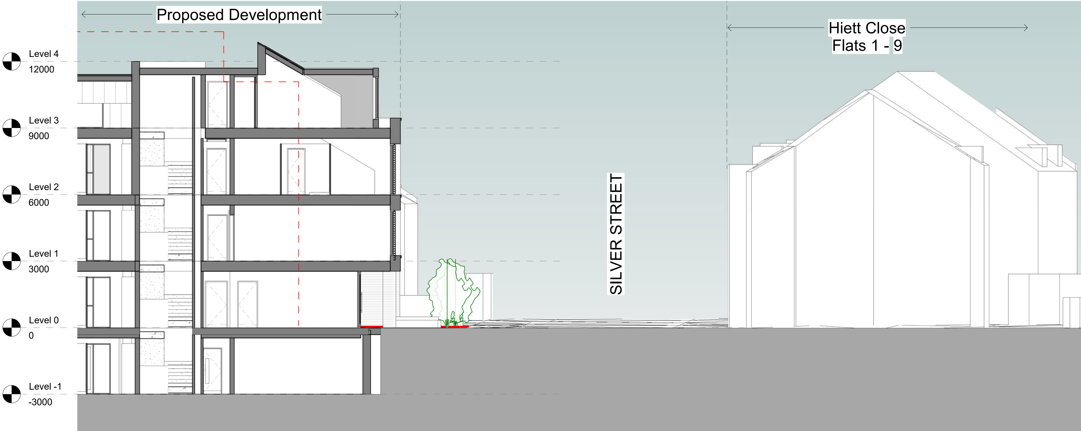
Section EE 1 : 100
