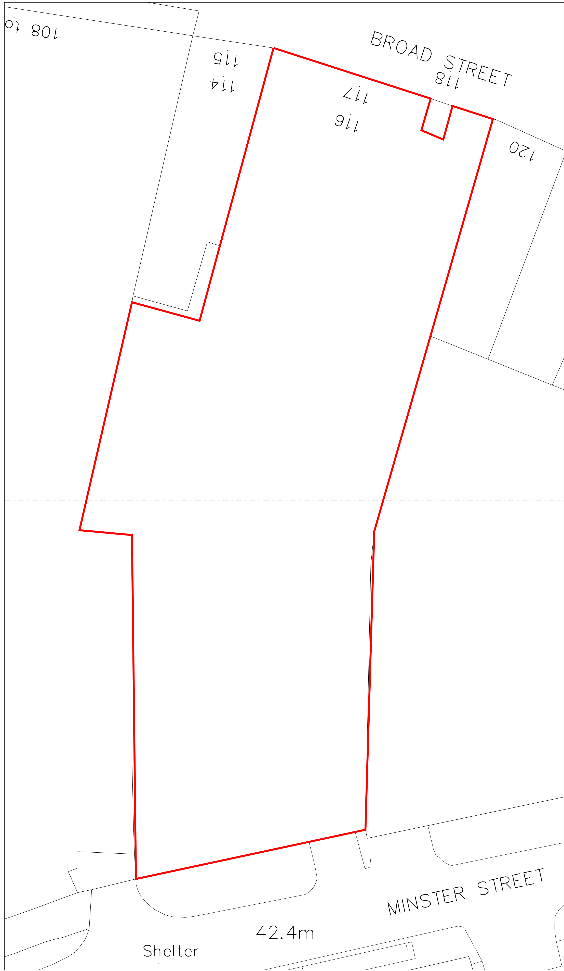
Site/Block Plan 1:200
