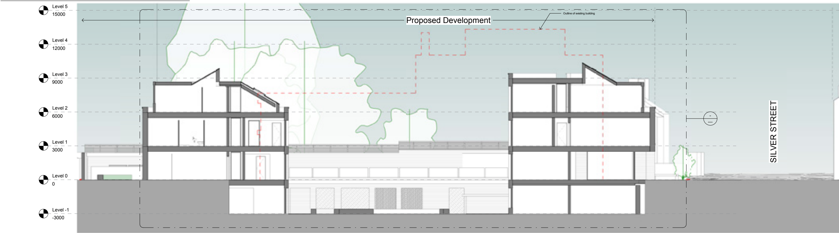
Section DD 1 : 100
