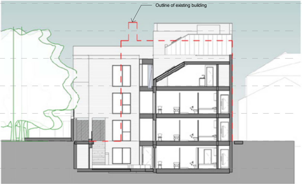
Section BB 1 : 200
