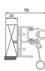
Jamb Detail
