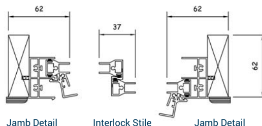
Jamb Detail
