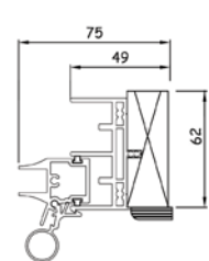
Jamb Detail
