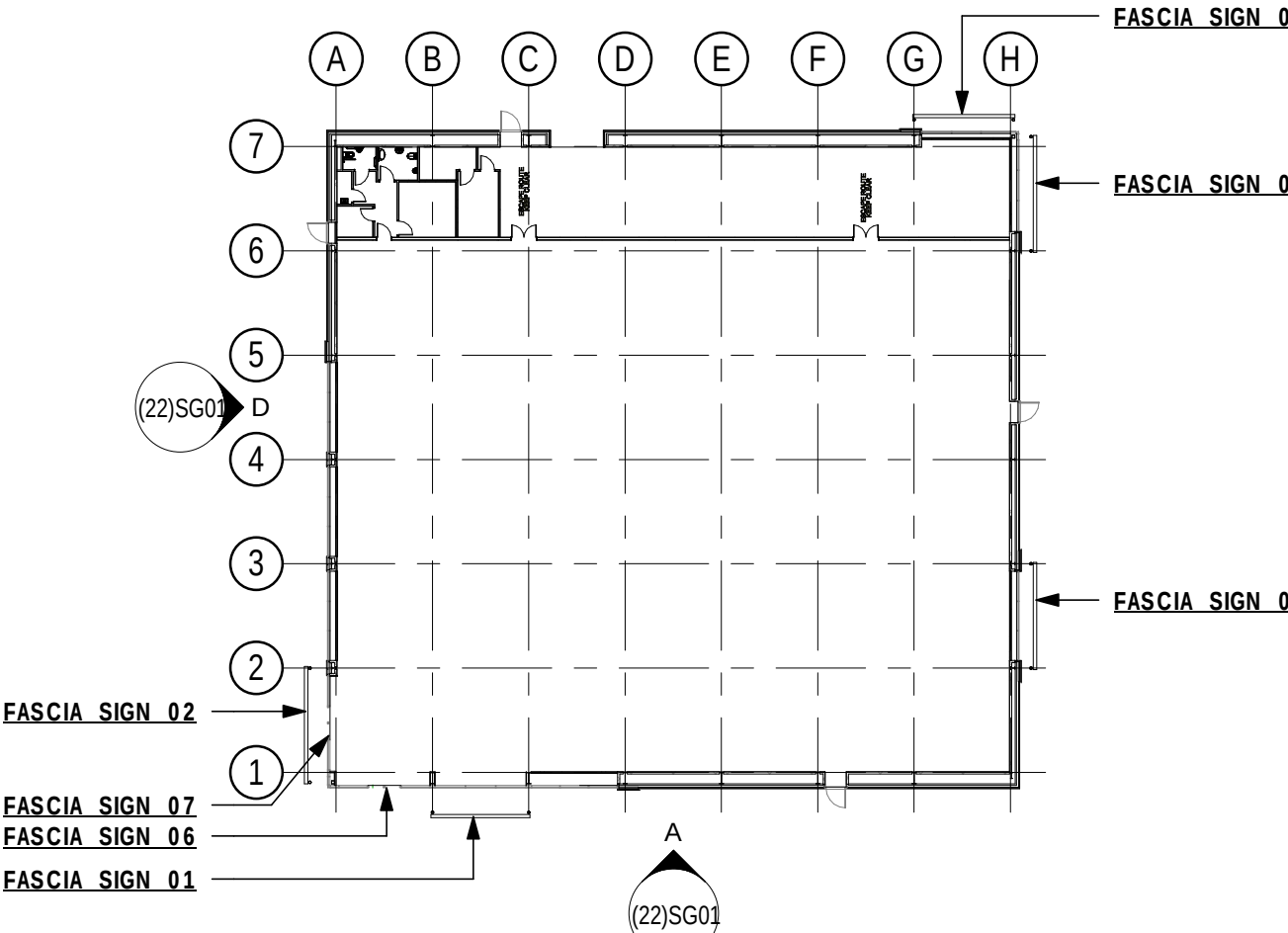
KEY PLAN 1 : 500
