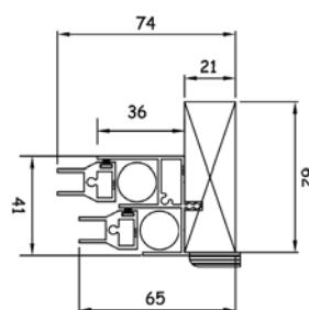
Jamb Detail
