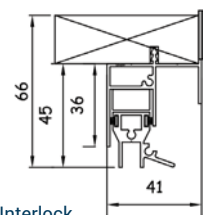
Interlock
