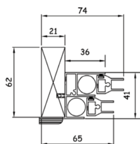
Jamb Detail
