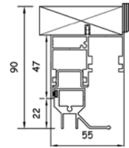
Interlock
