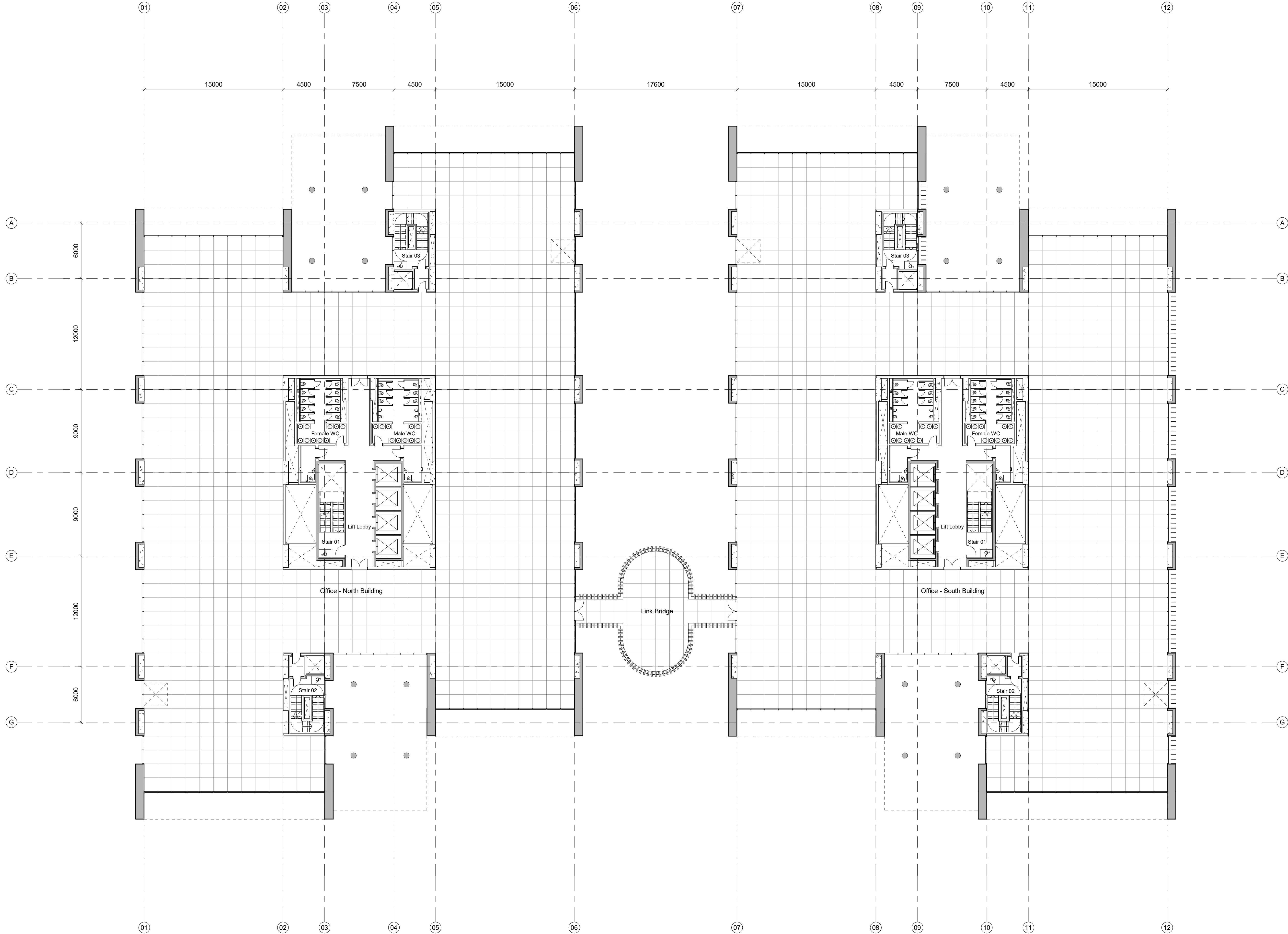
01 Level 03 1 : 200
