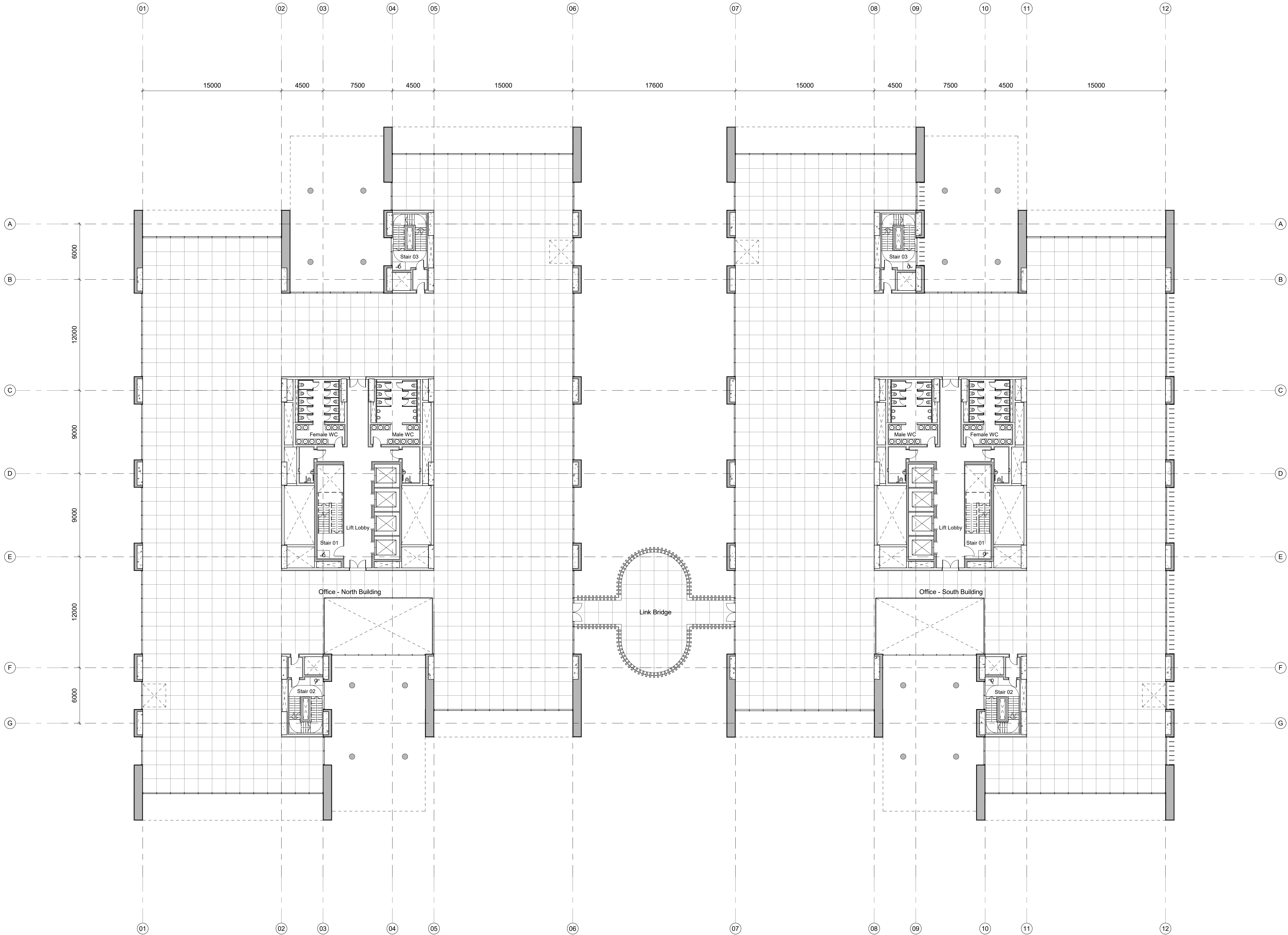
01 Level 01 1 : 200
