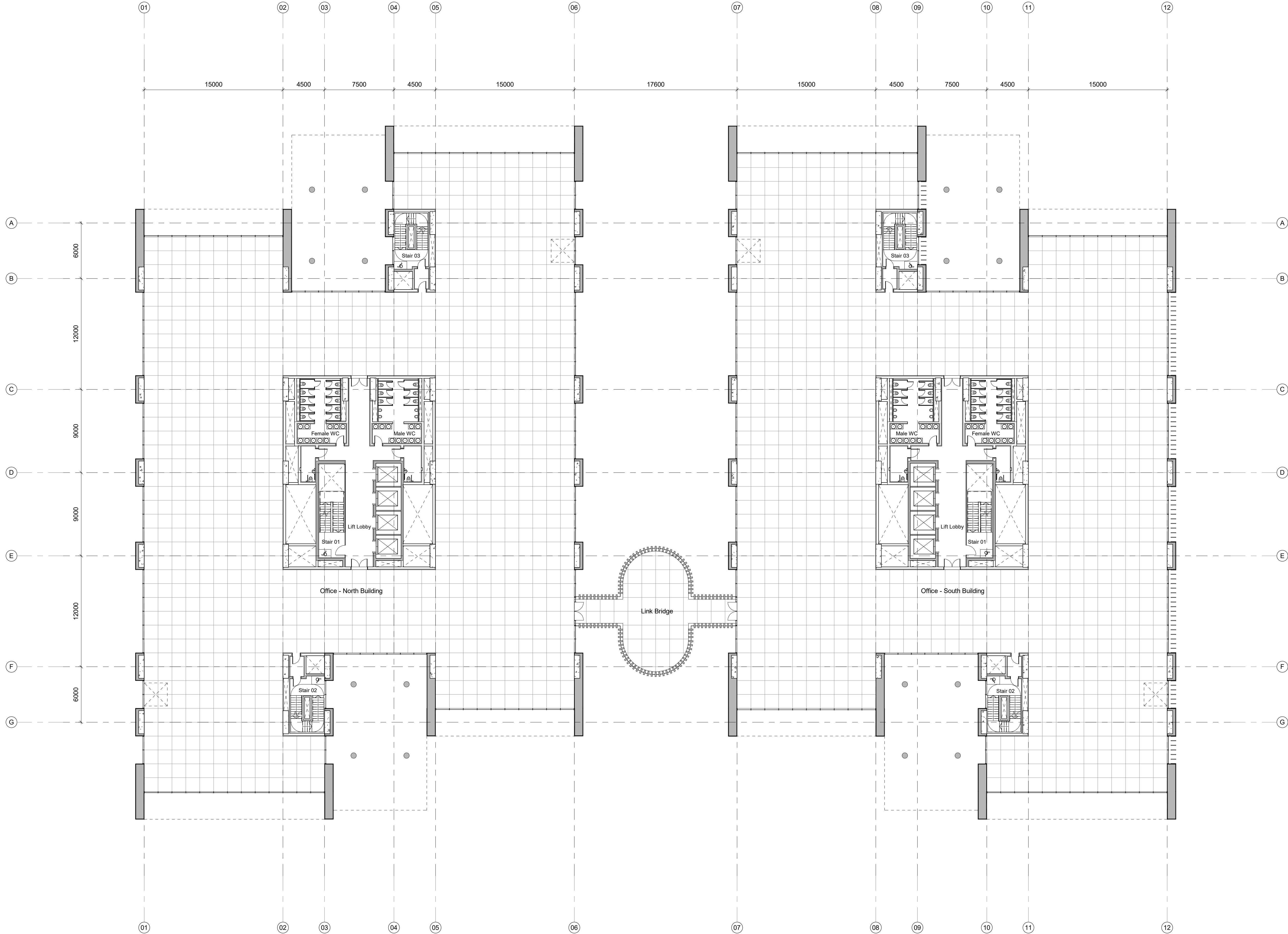
01 Level 02 1 : 200
