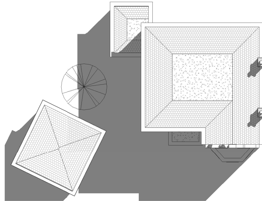
2 03. Roof plan 1 : 200
