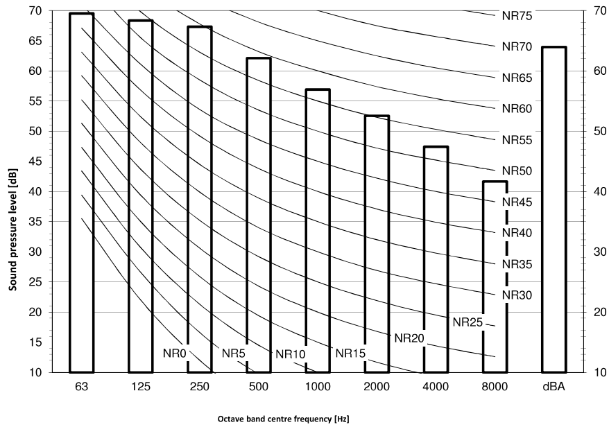
REYQ16T
