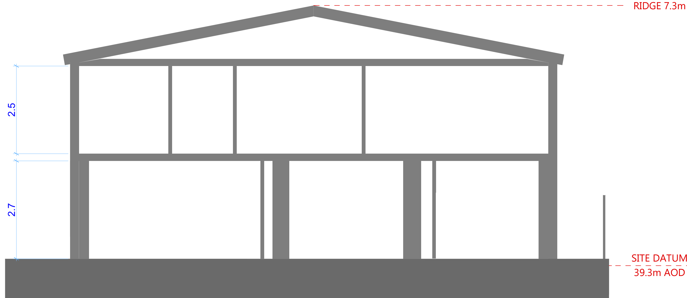
Section A-A Existing 1:50
