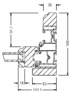
UPPER JAMB
