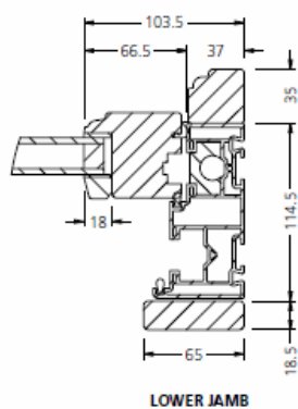
LOWER JAMB
