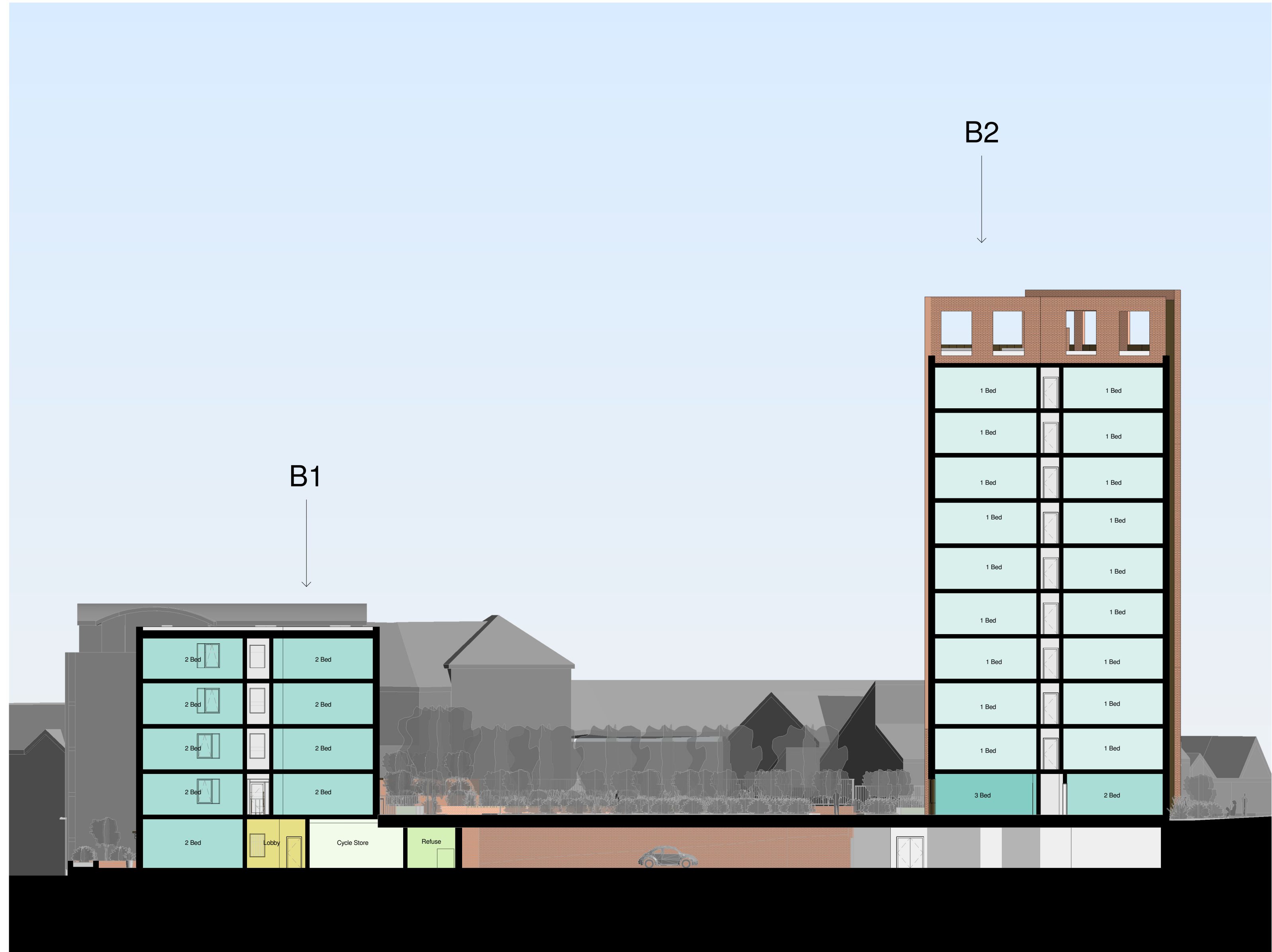
2 Section B-B 1 : 200
