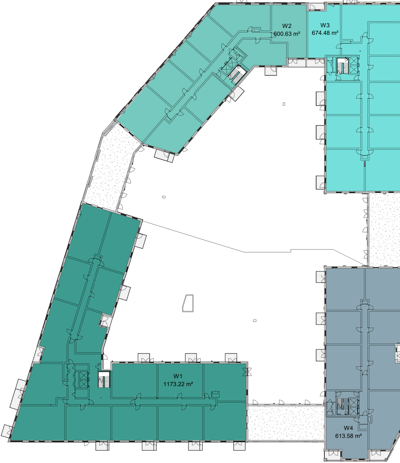
Level 3 1 : 500
