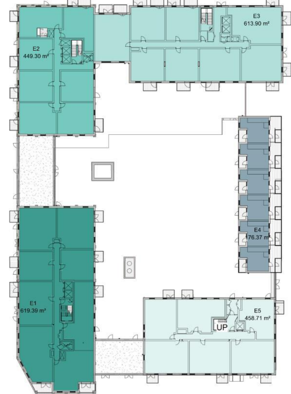
Level 3 1 : 500
