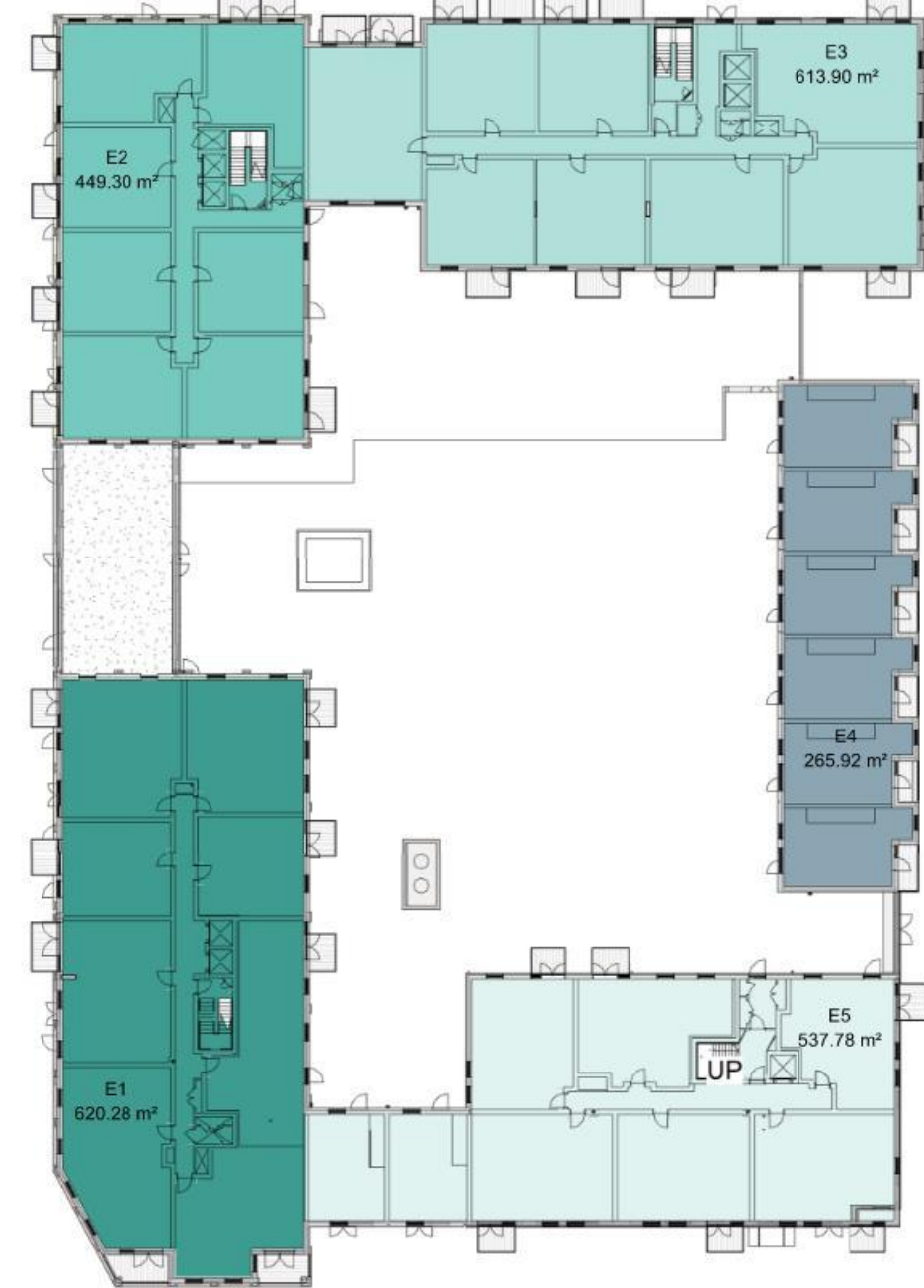
Level 2 1 : 500
