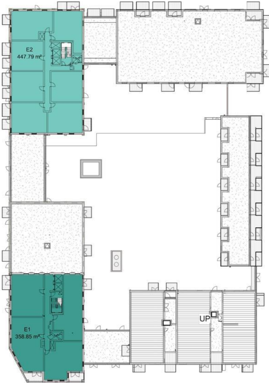
Level 7 1 : 500
