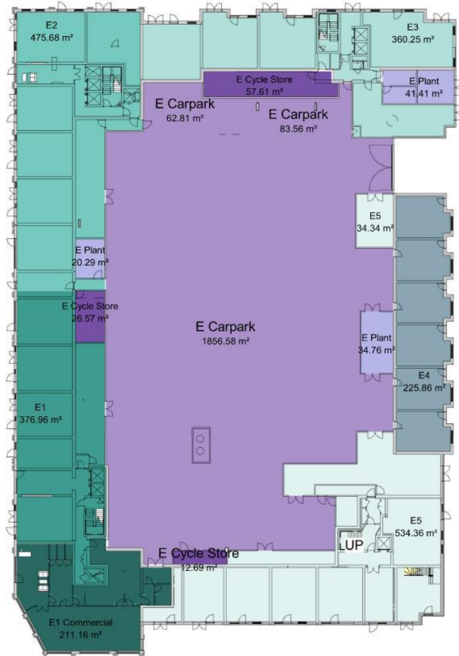
Level 0 1 : 500
