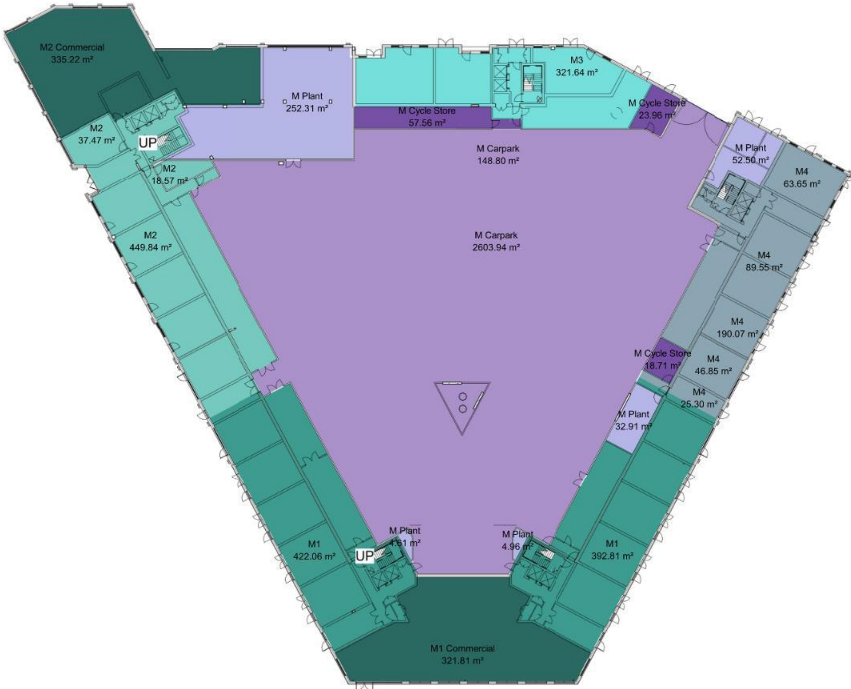
Level 0 1 : 500
