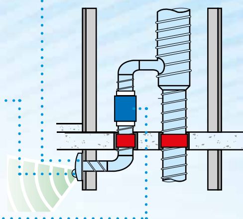
NRG Control Grille/Damper (optional).
