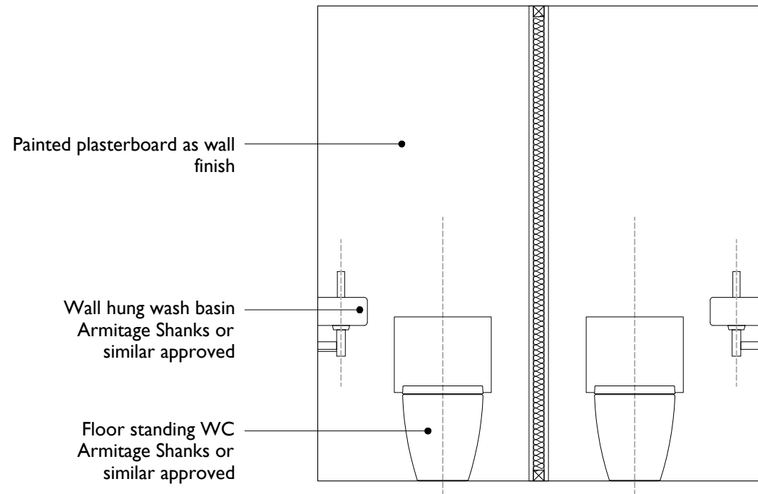
02 Elevation 01
