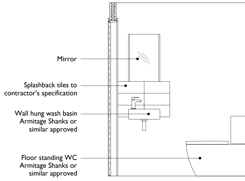
07 Elevation 06
