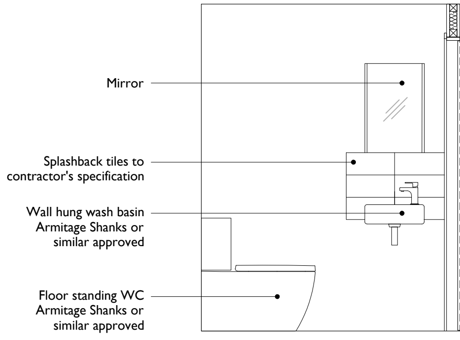
03 Elevation 02
