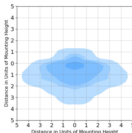
Isoilluminaance Plot
